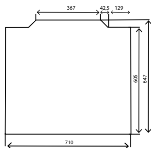
SKLENĚNÁ/PLECHOVÁ PODLOŽKA
