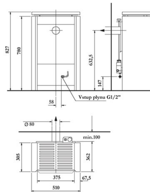
Pohled shora bez krycího kamene.
